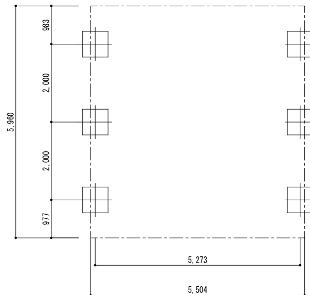
■ 基礎配置図
